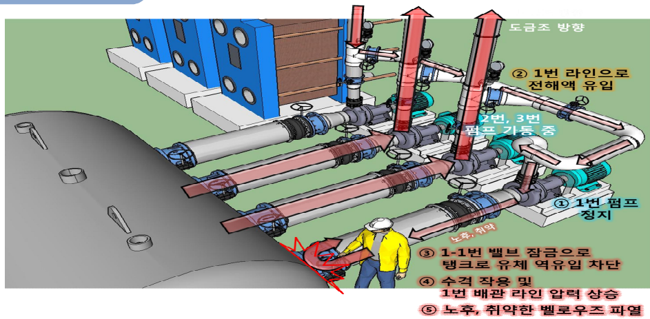
재해 상황 추정도
