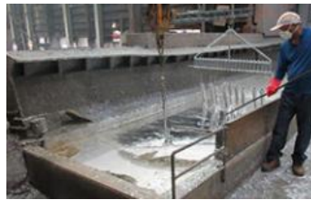
5 도금조 슬러지 제거
