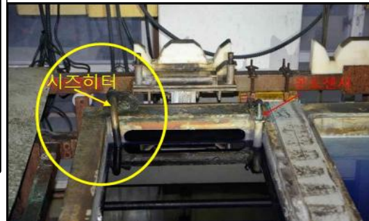
○ 시즈히터(Sheath Heater) - 탈지조 내의 온도를 55℃로 가열하기 위한 히터
