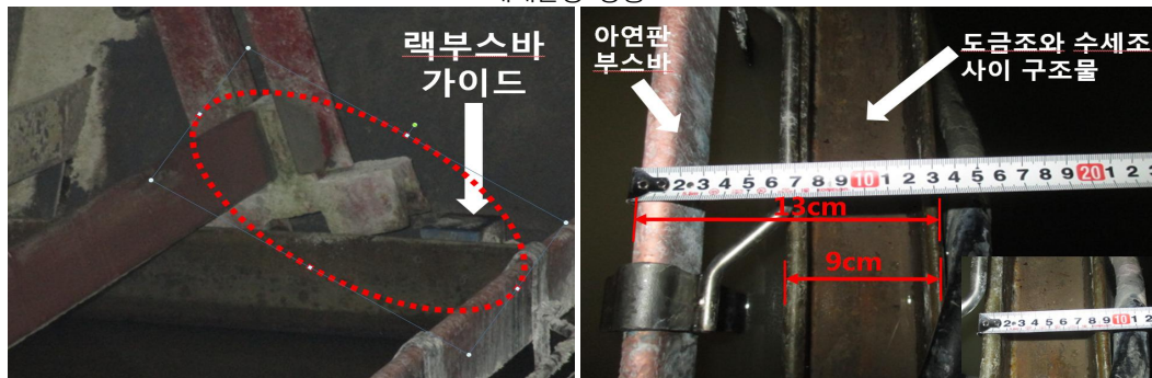
재해자 밟고 이동한 구조물
